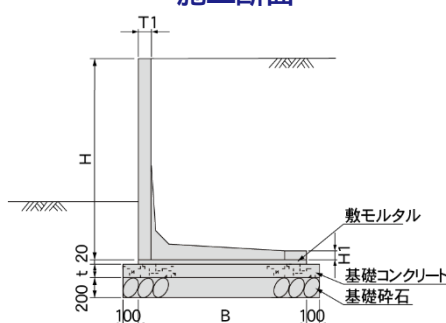
施工断面
