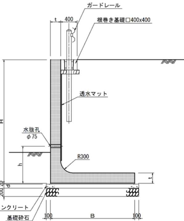
施工断面
